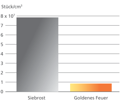
Feinpartikelgehalt der Rauchgase (red. O 2 =13%)**
