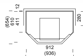
Höhe 1824 mm
