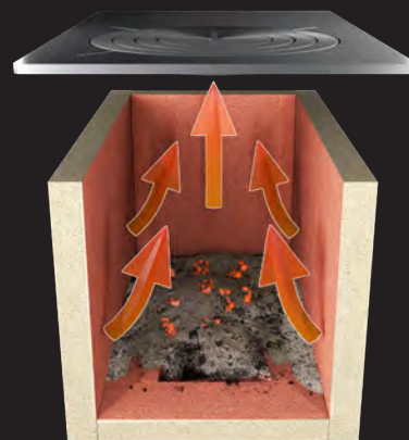
Phase 2: Konstante und allmähliche Freisetzung von Wärme, auch wenn das Feuer bereits erloschen ist
